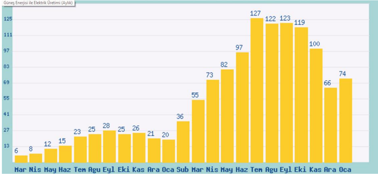
Şekil 6: 2017 yılı Ocak ayı ve öncesi 24 aylık dönemde güneş enerjisi ile gerçekleştirilen elektrik üretimi (Kaynak: TEİAŞ)
