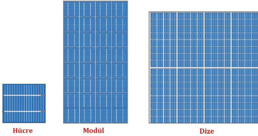
Şekil 29: Hücreler modülü, modüller dizeyi oluşturur [64]
