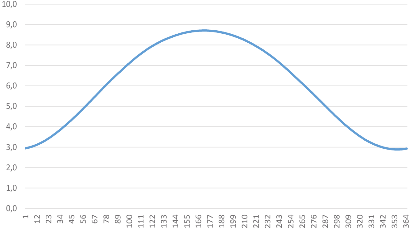
Şekil 64: Osmaniye açık gökyüzü teorik güneş ışıması potansiyeli, kWh/gün [96]
