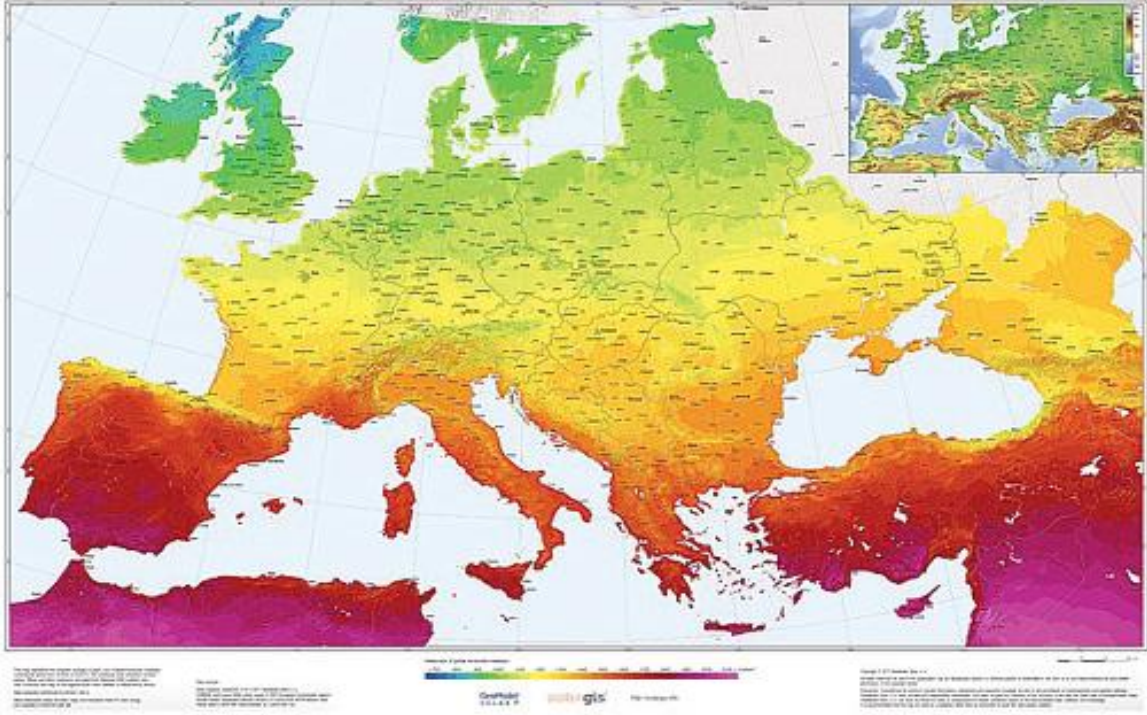
Şekil 52: SolarGIS Avrupa ve Türkiye güneş ışıma potansiyeli [88]
