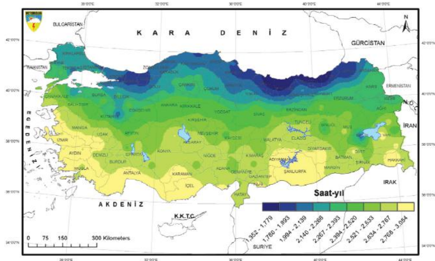
Şekil 57: MGM Türkiye yıllık toplam güneşlenme süreleri [94]
