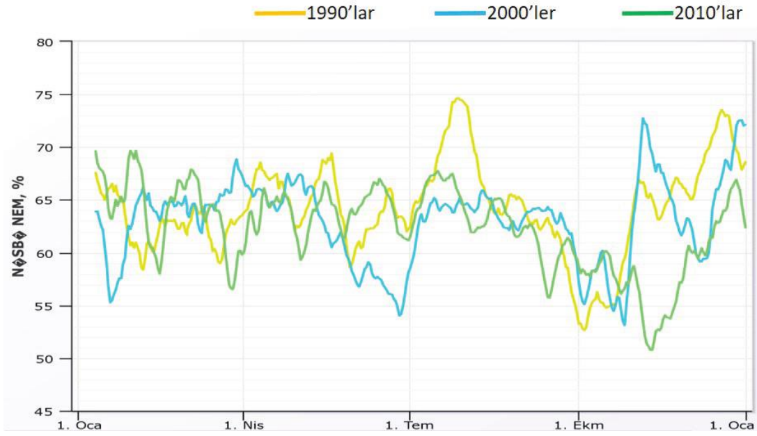
Şekil 17: Osmaniye nispi nem 3 on yıl
