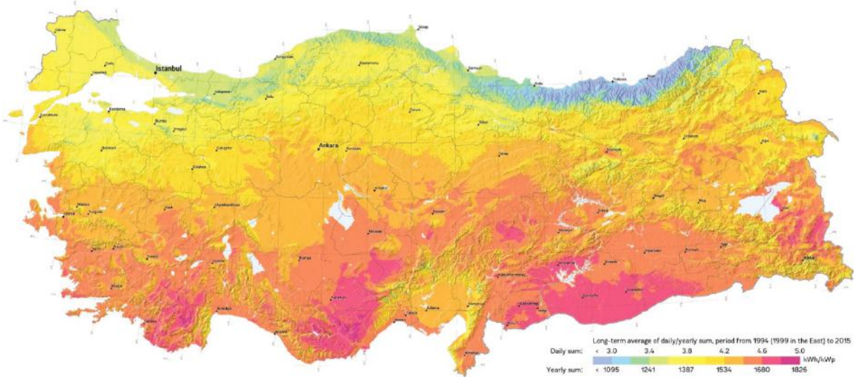
Şekil 54: Global Solar Atlas Türkiye güneş enerjisi potansiyeli
