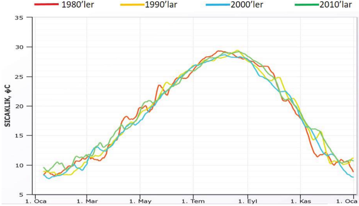
Şekil 15: Osmaniye ortalama sıcaklık 4 on yıl
