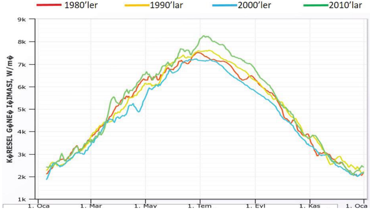
Şekil 26: Osmaniye maksimum güneş ışıması 4 on yıl
