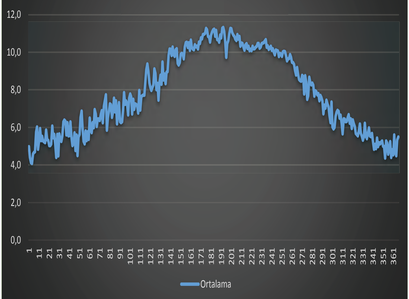
Şekil 65: Osmaniye güneşlenme süresi ölçümleri, Saat/gün (1985-2015)
