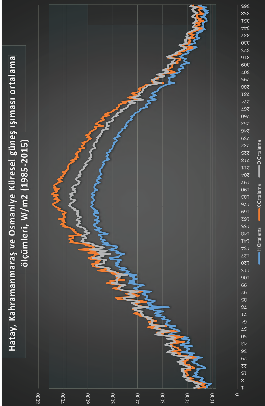
Şekil 60: TR63 Bölgesi Küresel güneş ışıması ortalama ölçümleri
