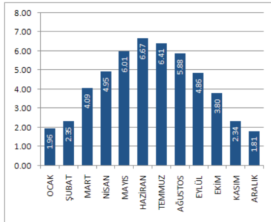
Şekil 46: GEPA Osmaniye ay bazlı günlük küresel radyasyon (güneş ışıması), 4 \text{ kWh/m}^2
