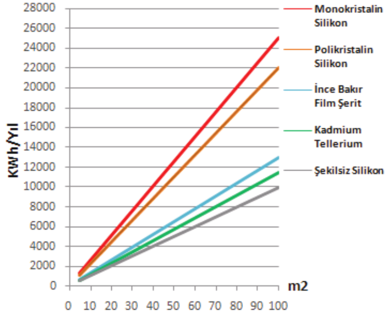
Şekil 34: FV yapıların birim alanda yıllık elektrik üretebilme kapasiteleri, GEPA [3]
