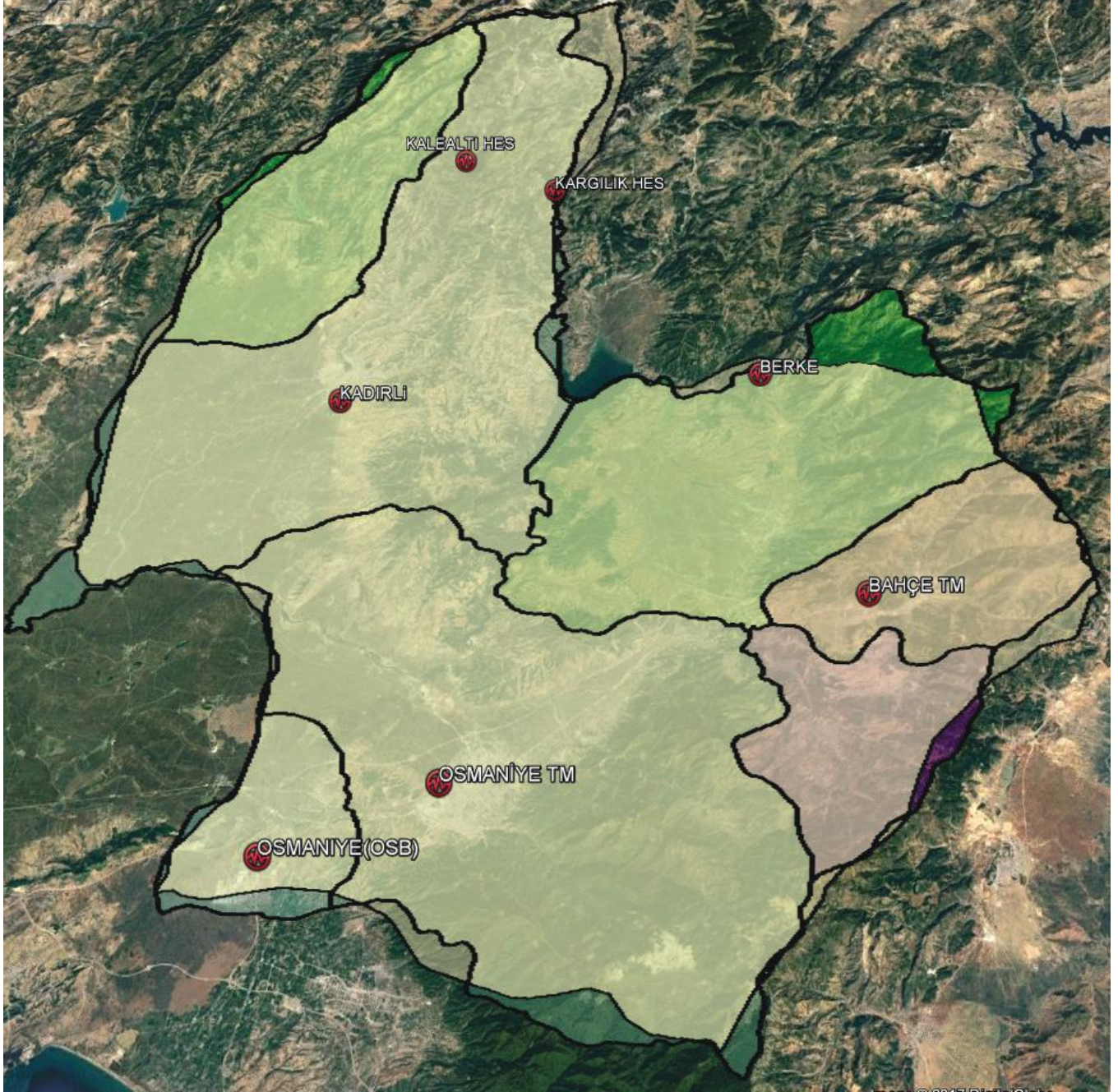
Şekil 68: Osmaniye TEİAŞ trafo merkezleri
