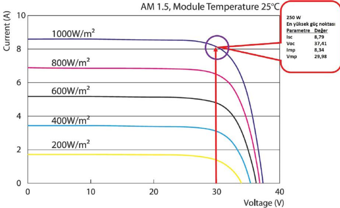
Şekil 32: Bir hücrenin örnek akım-gerilim grafiğı
