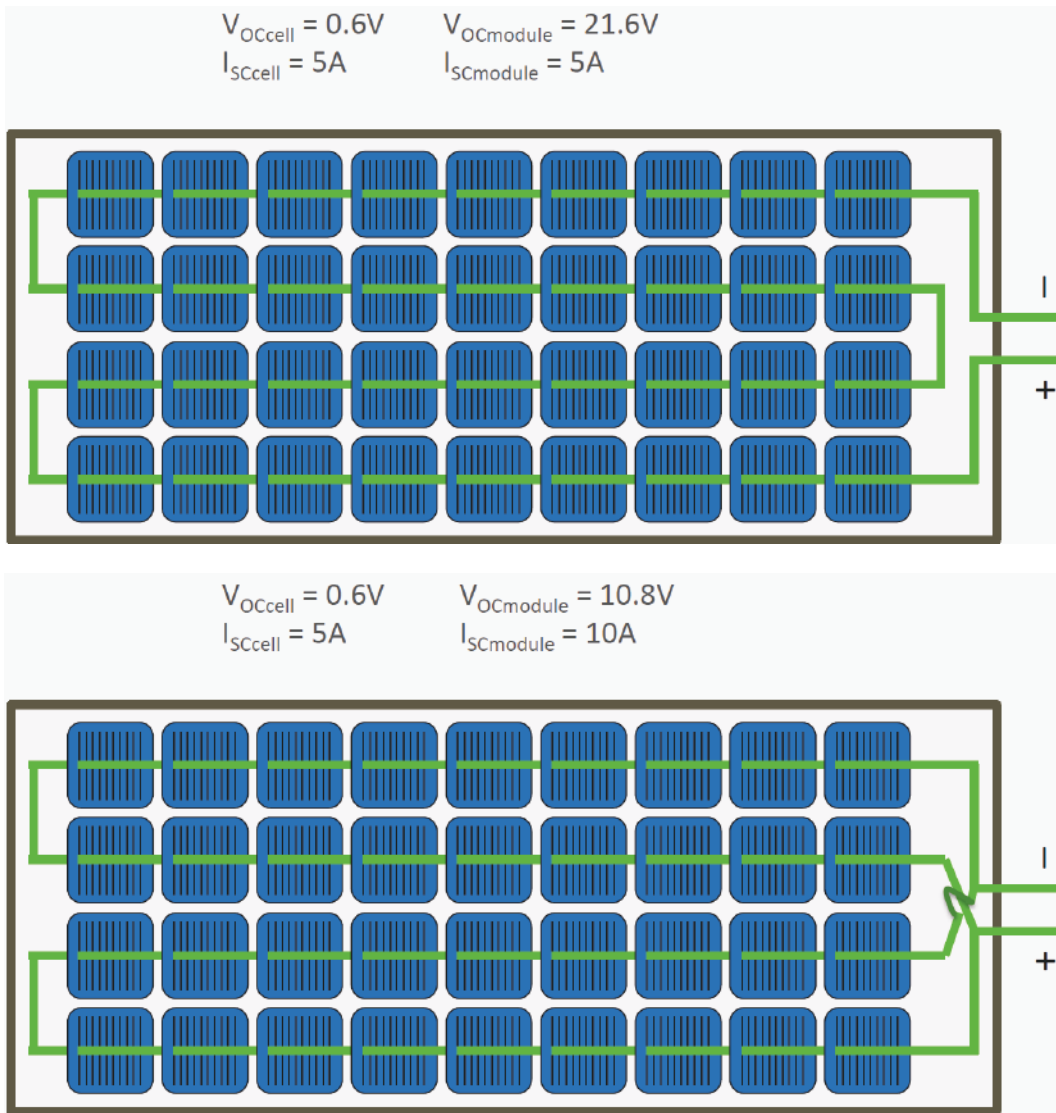
Şekil 31: FV modül hücrelerinin seri ve paralel bağlantı ile akım gerilim ayarlaması [66]
