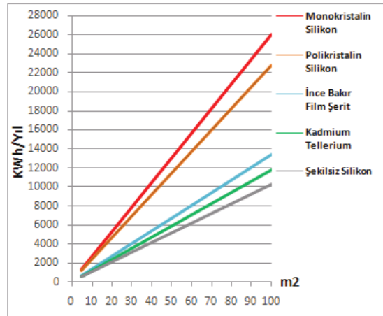
Şekil 47: GEPA Osmaniye PV Tipi-Alan-Üretilebilecek Enerji ( \text{kWh-Yıl} )
