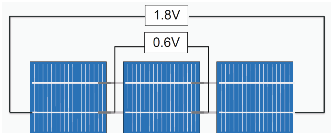
Şekil 30: FV hücrelerin seri bağlantısı
