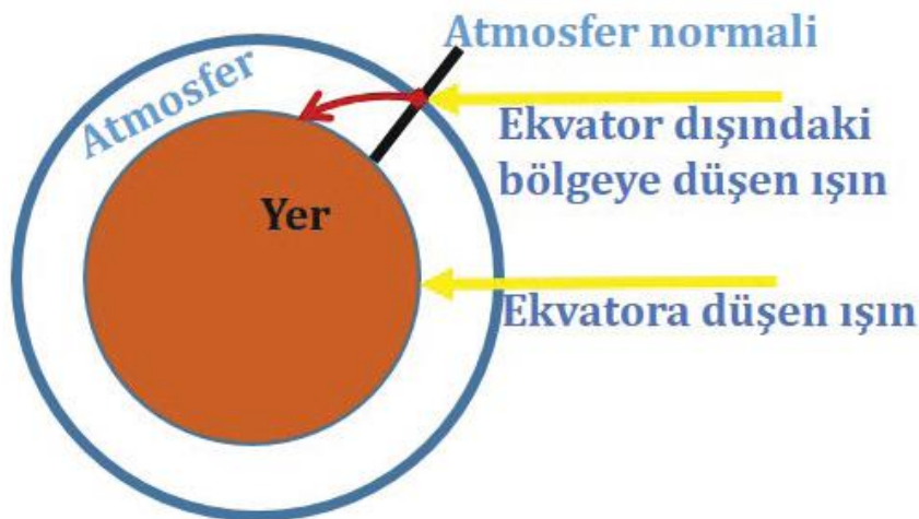
Şekil 39: Işınların atmosferde izlediği Yol
