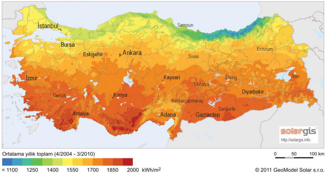
Şekil 53: SolarGIS Türkiye küresel yatay radyasyon (güneş ışıması) haritası [88]
