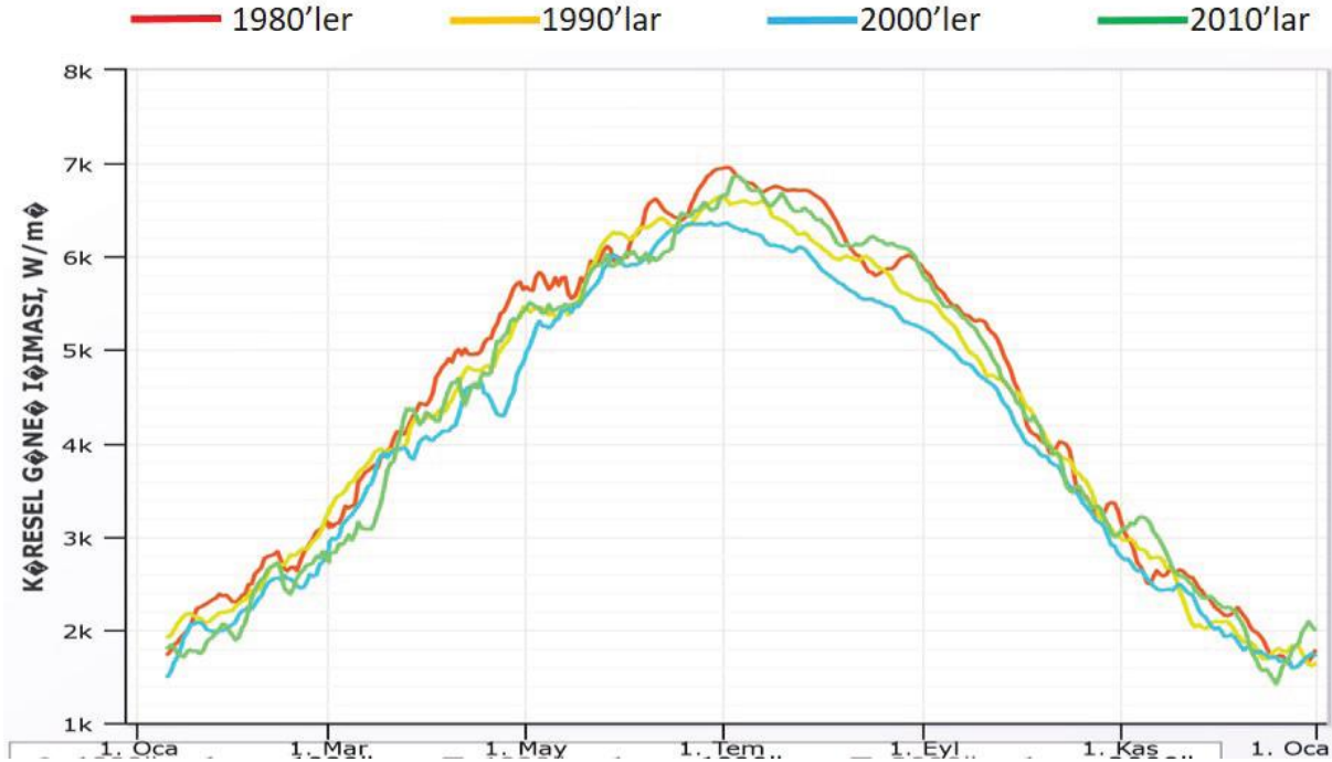
Şekil 25: Osmaniye ortalama güneş ışıması 4 on yıl
