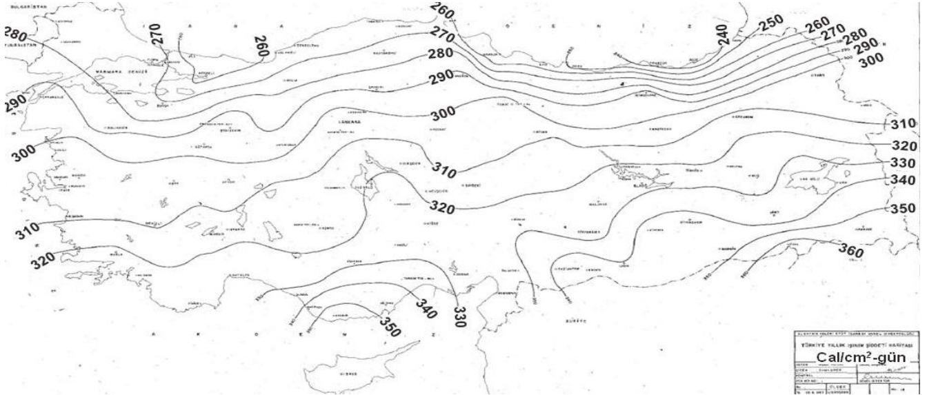
Şekil 56: Türkiye yıllık ışıma şiddeti haritası, cal/cm 2 -gün (Kaynak: DMI) [79]
