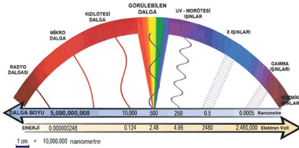
Şekil 27: Elektromanyetik spektrum
