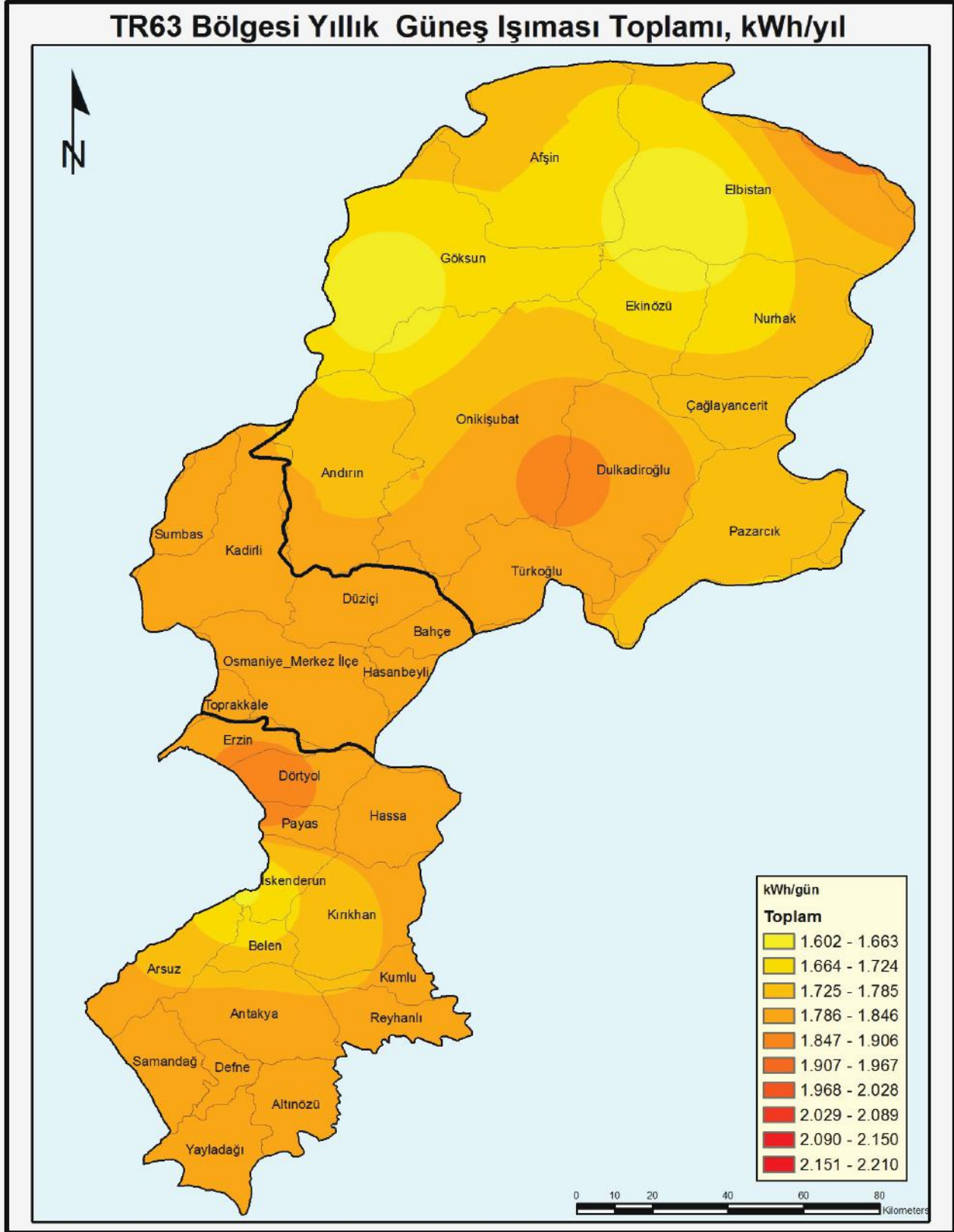
Şekil 72: TR63 Bölgesi yıllık güneş ışıması değerleri haritalaması
