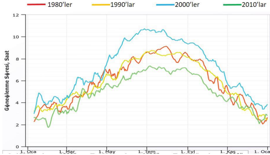
Şekil 23: Osmaniye ortalama güneşlenme süresi 4 on yıl
