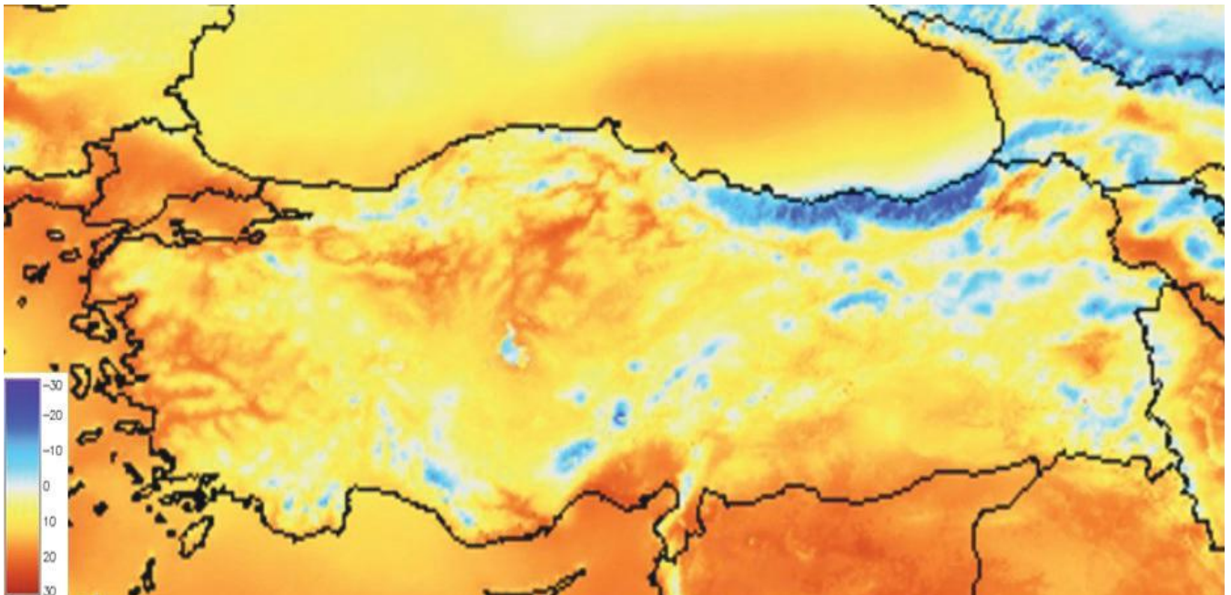
Şekil 49: PVGIS-3 ve PVGIS-CMSAF arasındaki radyasyon değişimi, Türkiye
