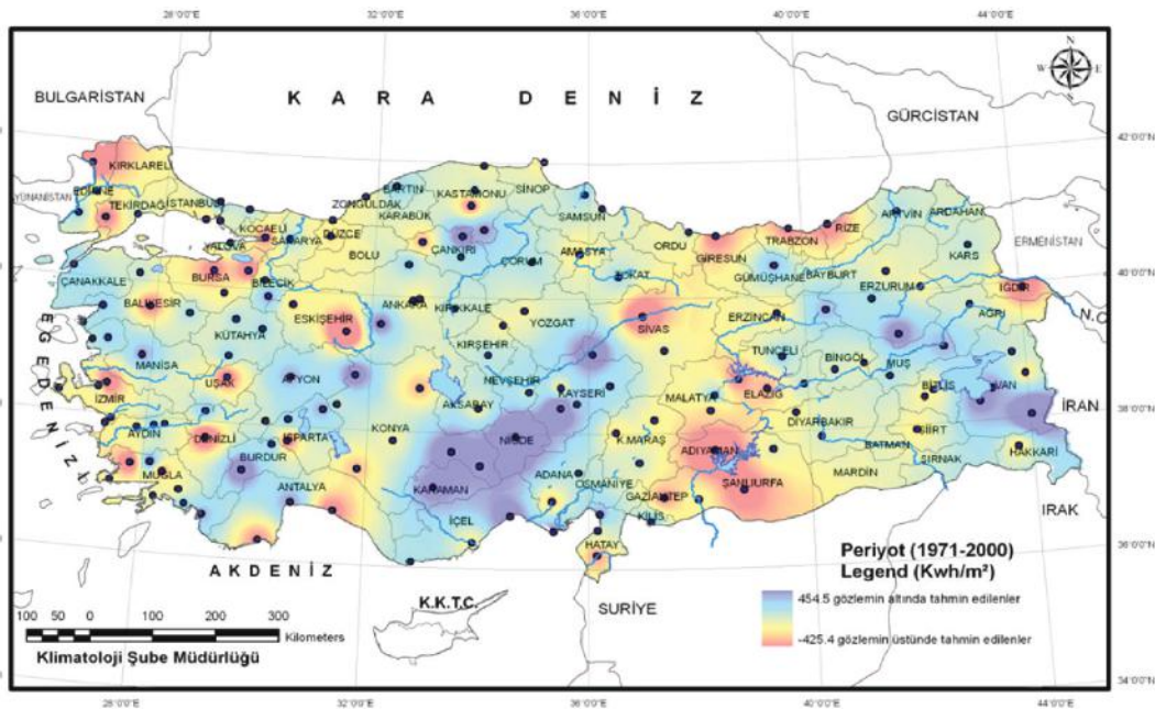
Şekil 59: Gözlenen güneşlenme şiddeti ile GWR model çıktısı arasındaki kalıntı haritası [94]
