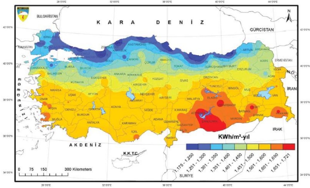
Şekil 58: MGM Türkiye yıllık toplam güneş radyasyonu (CAR modeline göre) [94]
