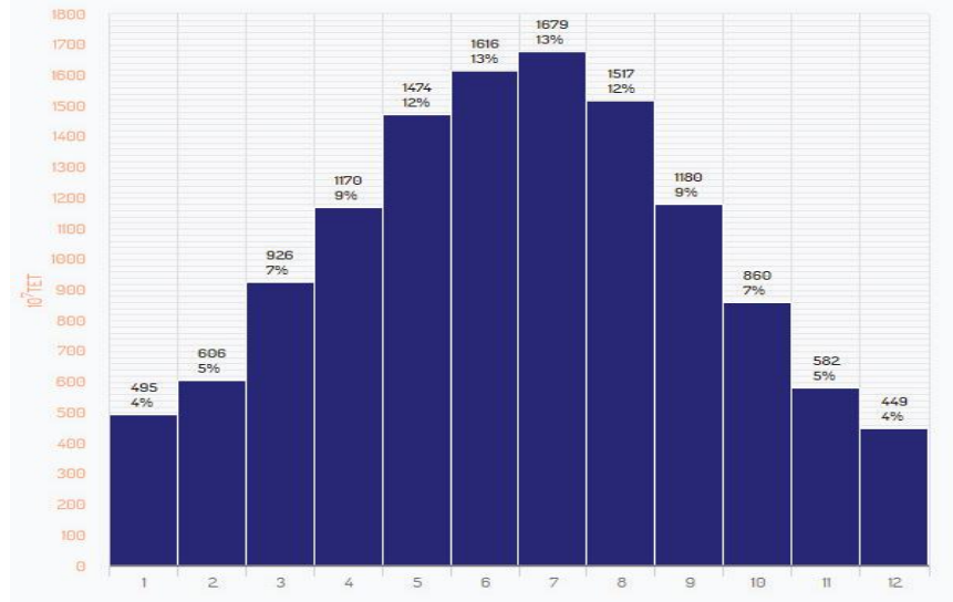
Şekil 55: Türkiye güneş enerjisi alansal ve zamansal dağılımı, 107 TET (Kaynak: DMİ) [79]
