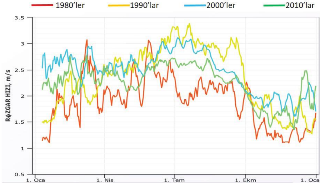
Şekil 20: Osmaniye maksimum rüzgar hızı 4 on yıl
