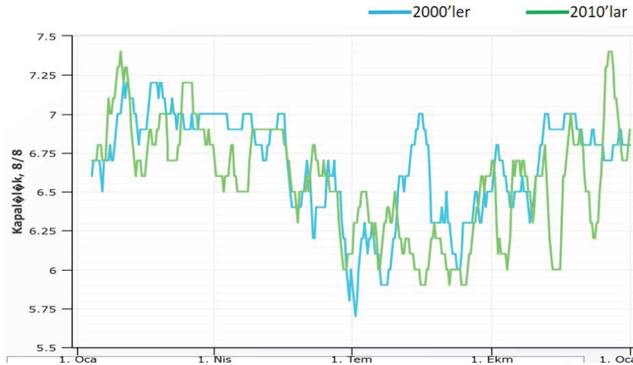
Şekil 22: Osmaniye maksimum kapallık 2 on yıl
