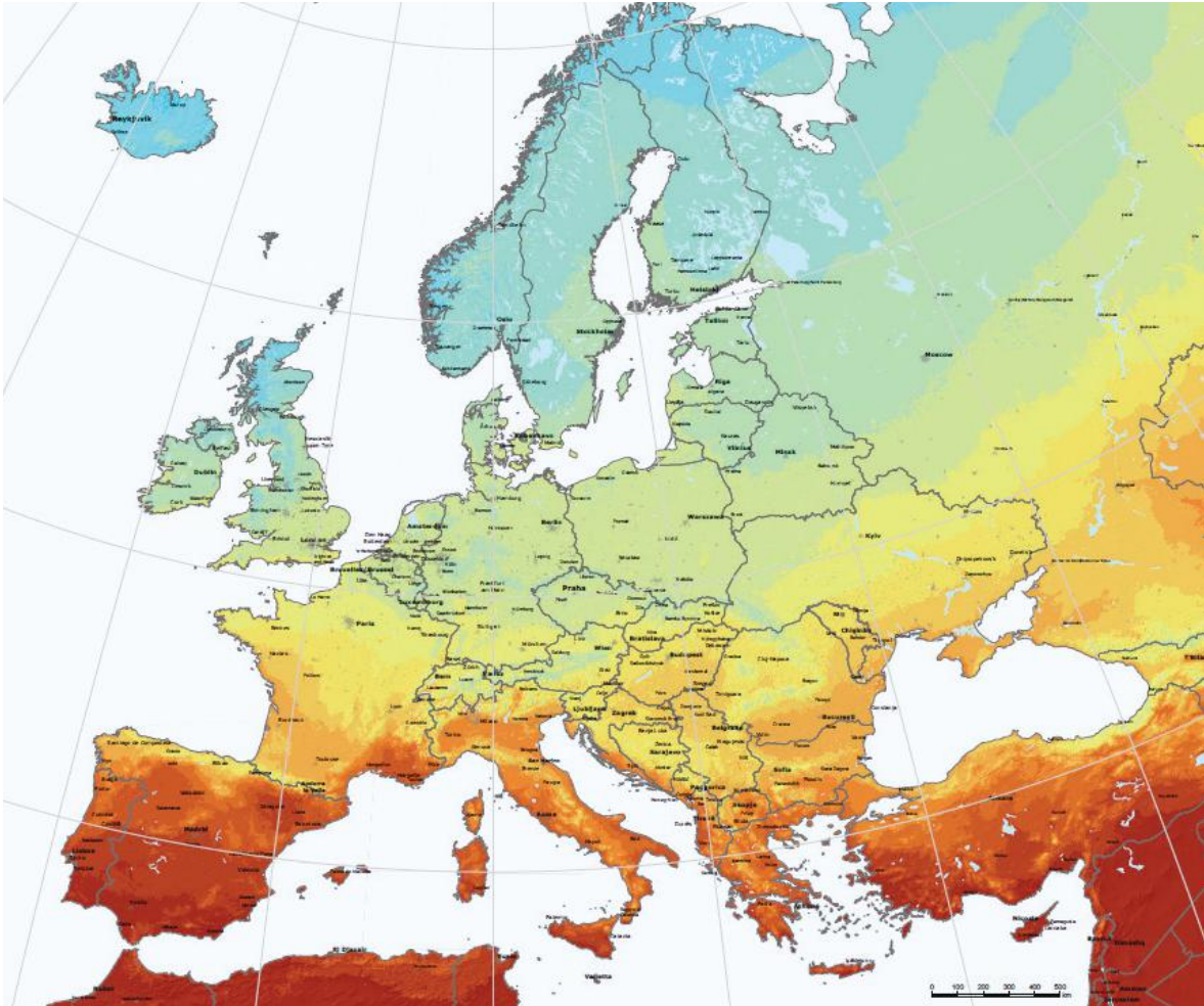
Şekil 50: PVGIS Avrupa güneş enerjisi potansiyel haritası [85]
