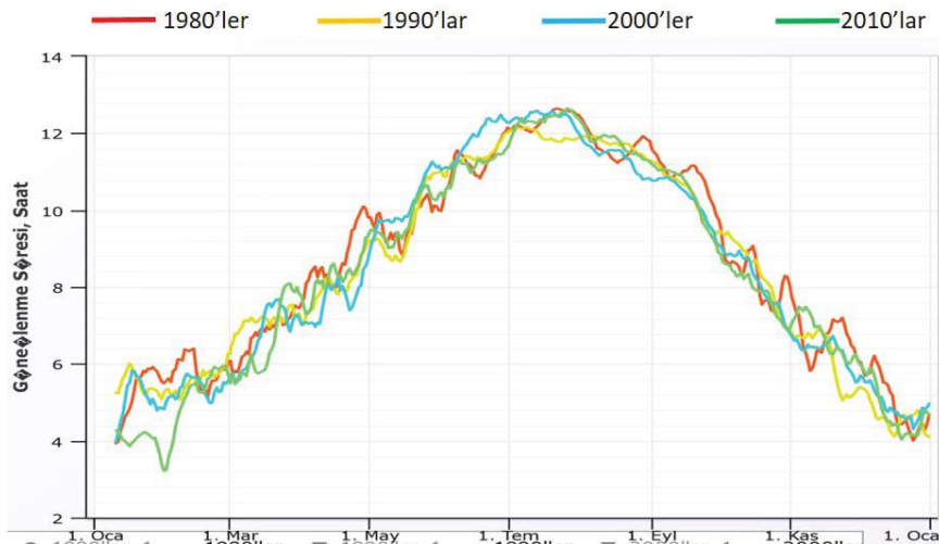
Şekil 24: Osmaniye maksimum güneşlenme süresi 4 on yıl
