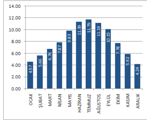
Şekil 45: GEPA Osmaniye ay bazlı günlük ortalama güneşlenme süreleri, saat
