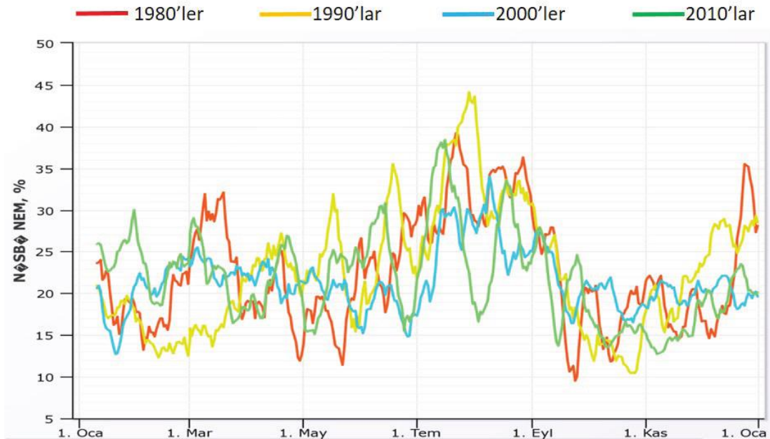
Şekil 18: Osmaniye minimum nispi nem 4 on yıl
