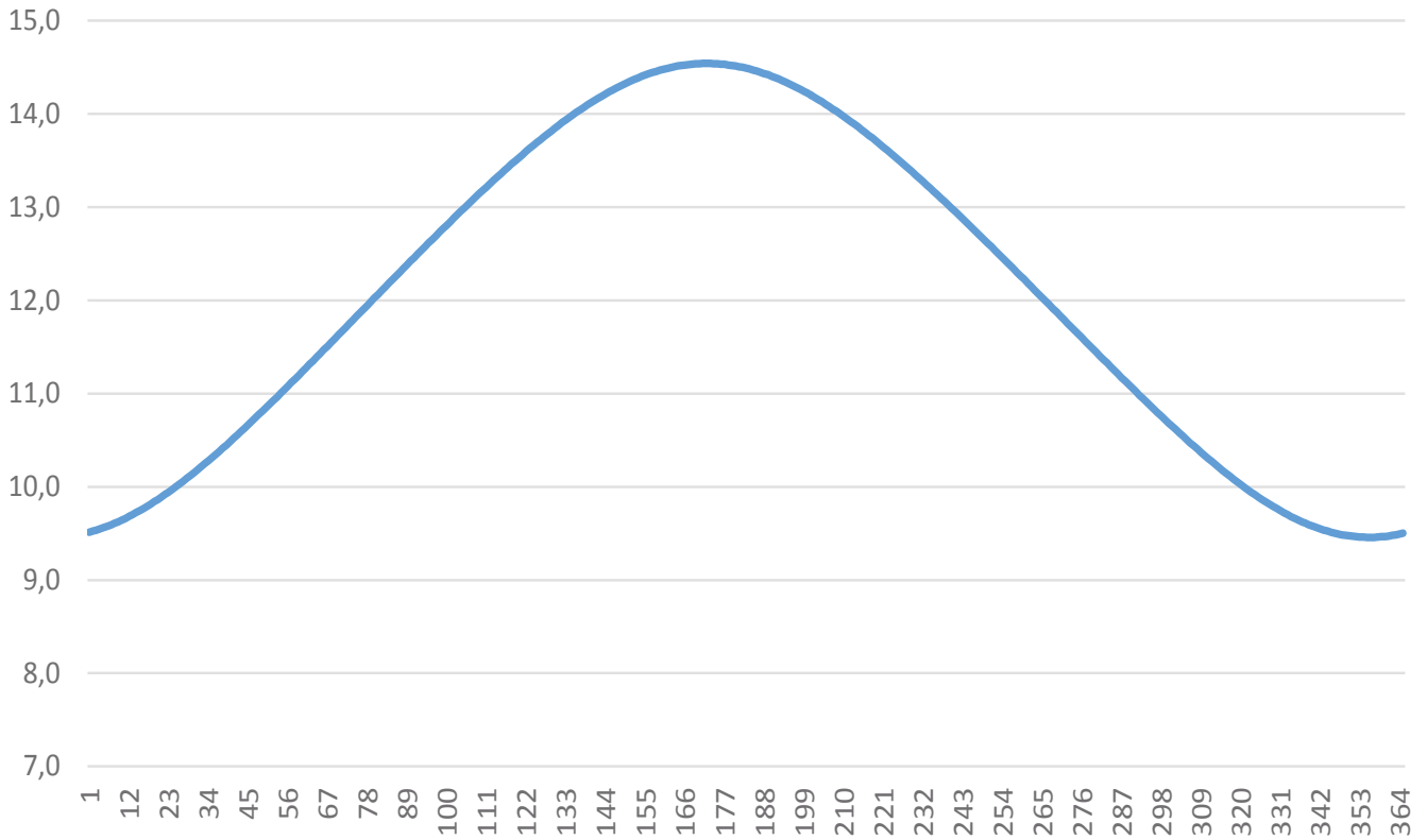
Şekil 63: Osmaniye açık gökyüzü teorik güneşlenme süresi, saat/gün [95]
