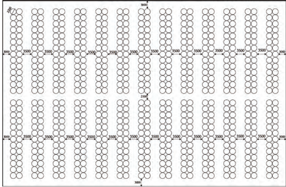
Resim 10. Zeytin Lisanslı Deposu Tank Yerleşimi
